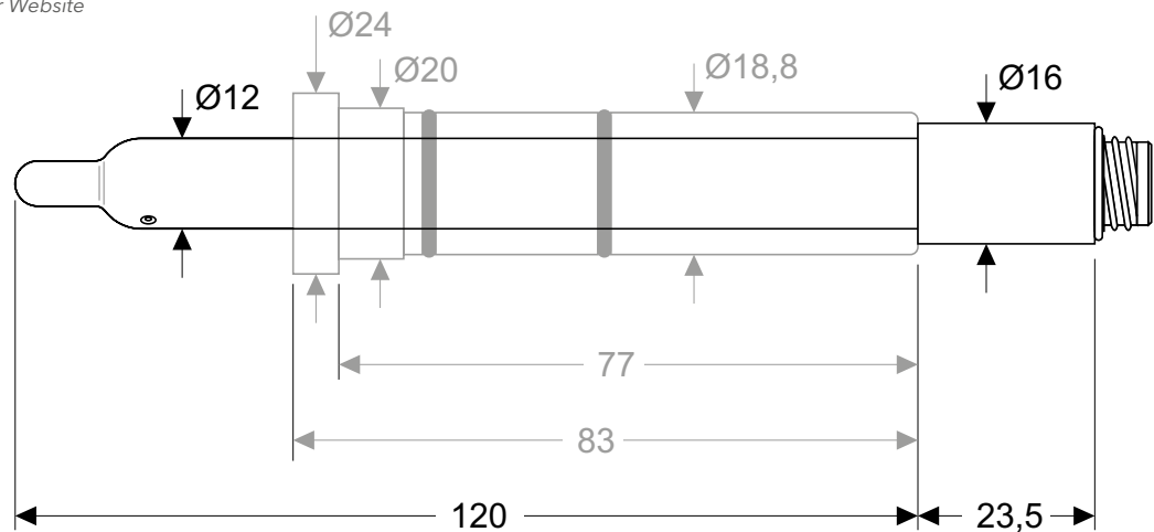
SensoLyt® Einstabmessketten
